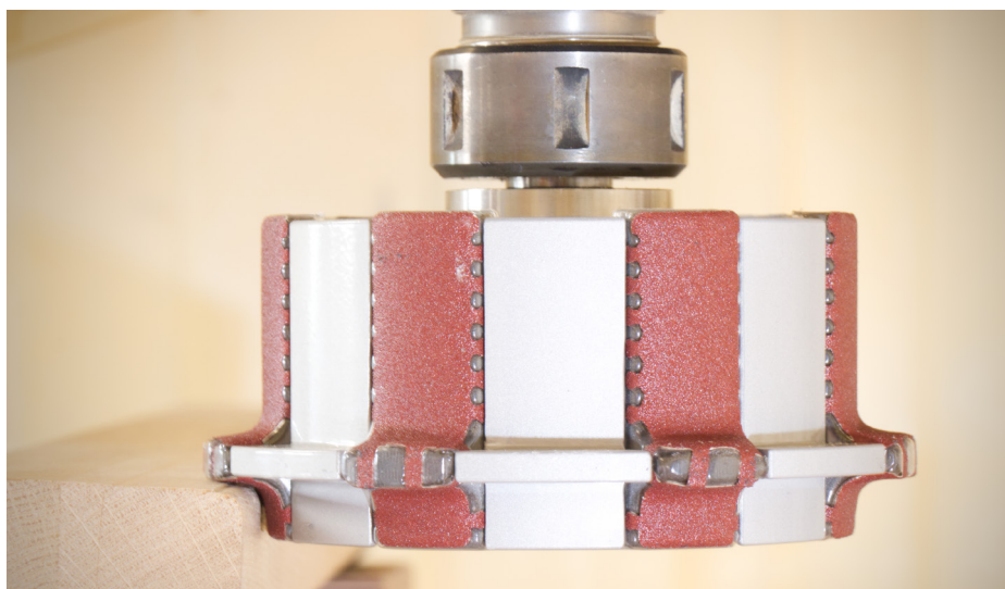
Kantenschleif-Variante: Radius.
